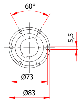
Flangia con fori di fissaggio FSB/25
